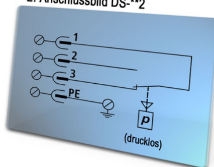
2. Anschlussbild DS-**2
